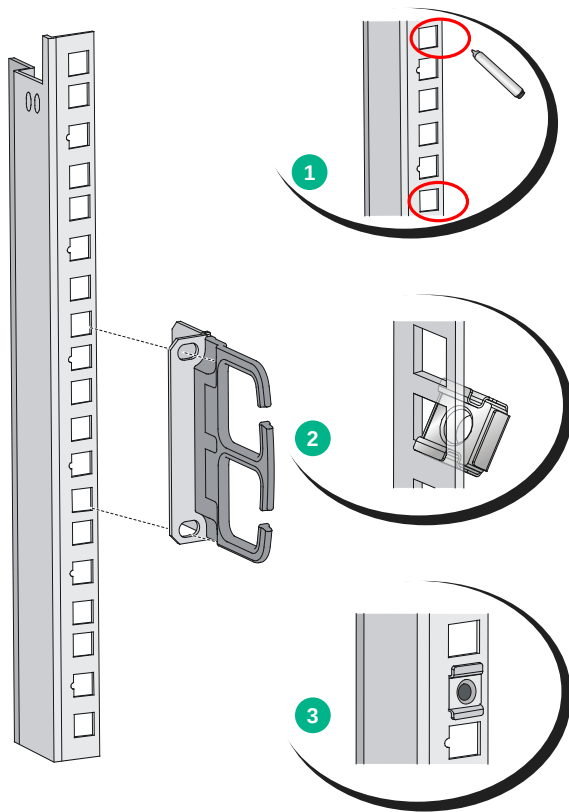
图2-3 安装浮动螺母
