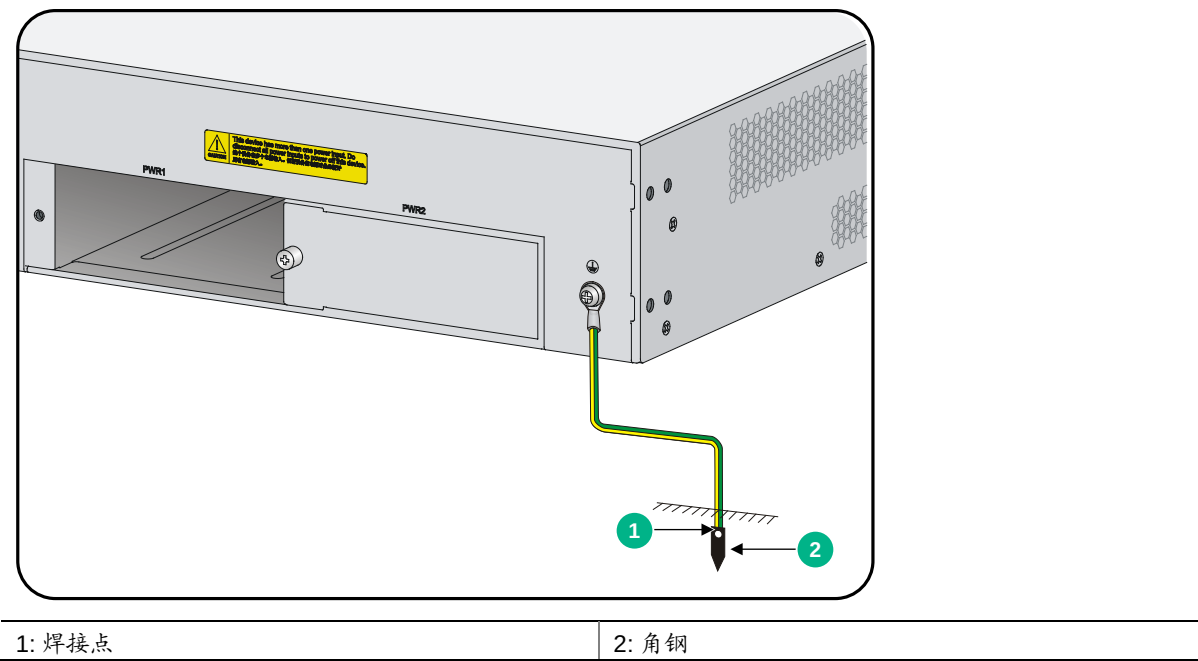
图2-9 机房附近允许埋设接地体时接地安装简图
