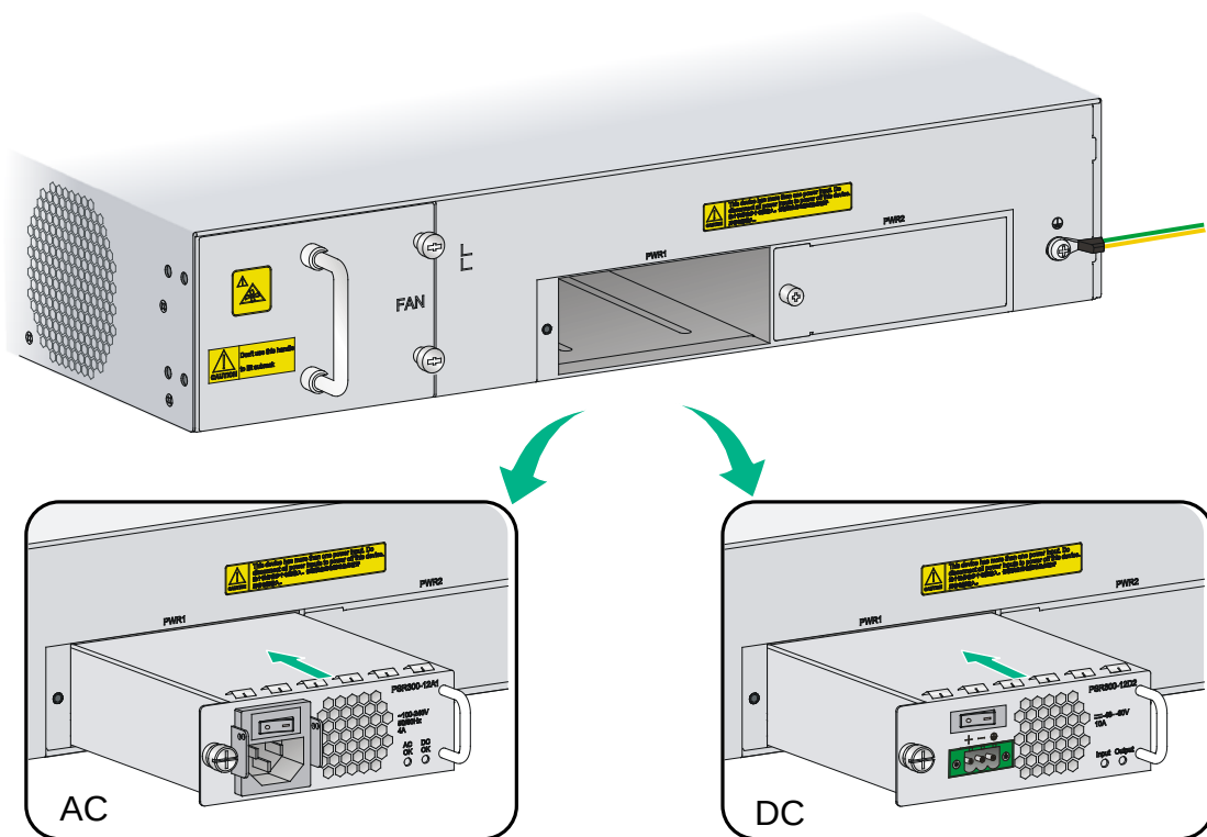
图2-10 安装电源模块
