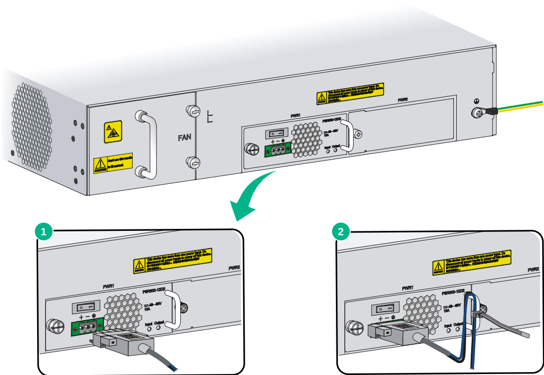
图2-16 连接直流电源线
