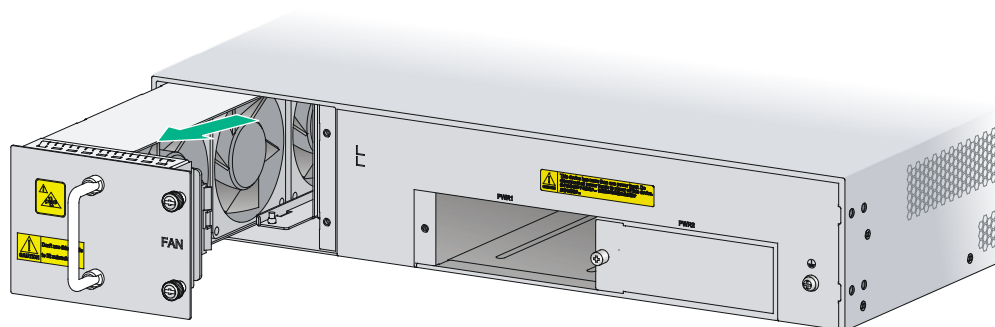
图4-5 将风扇框拉出风扇框插槽
