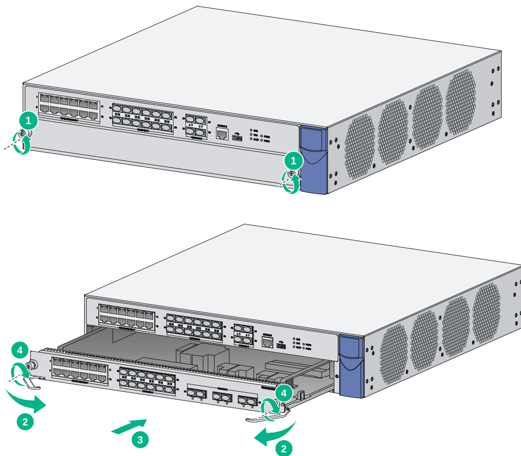
图2-11 安装接口模块
