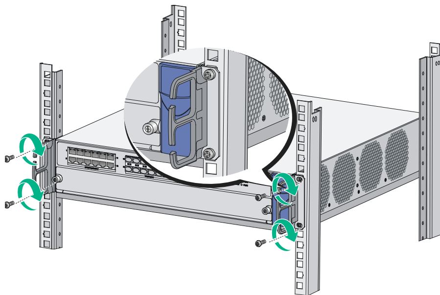
图2-6 固定设备到机柜
