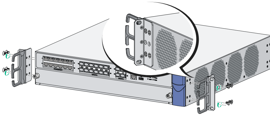
图2-4 安装挂耳到设备前面板的左、右两侧
