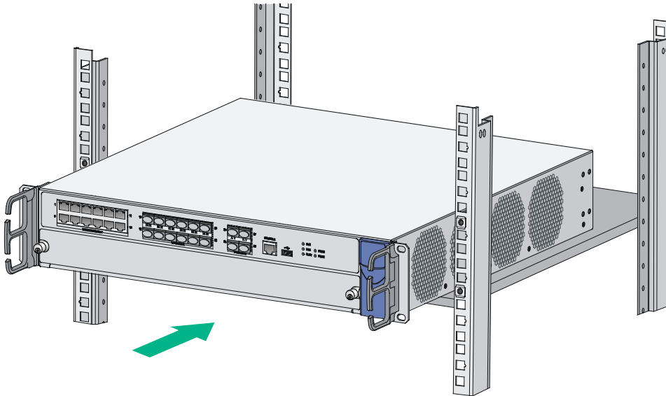
图2-5 安装设备到机柜
