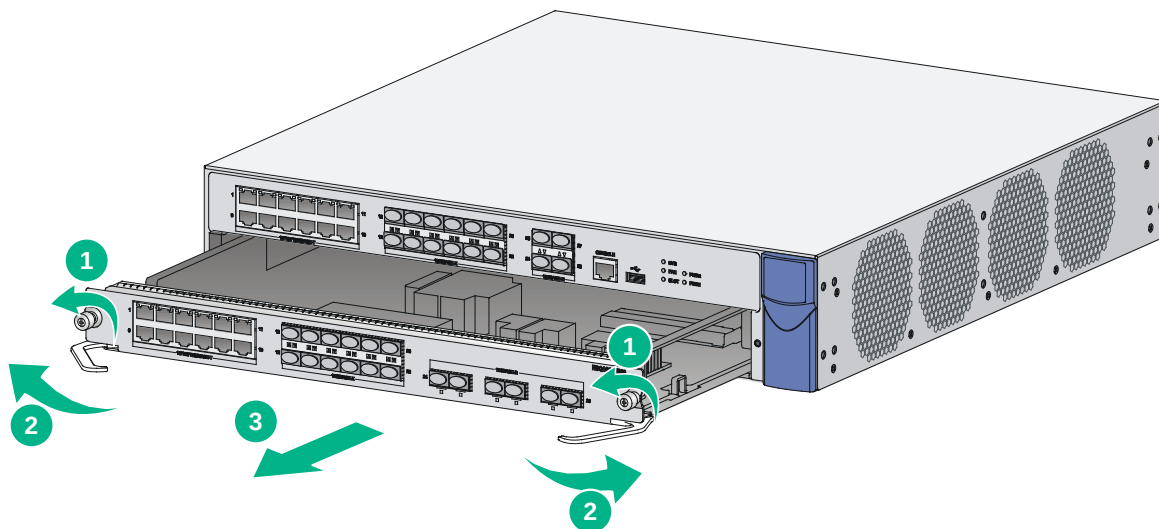
图4-2 拆卸接口模块
