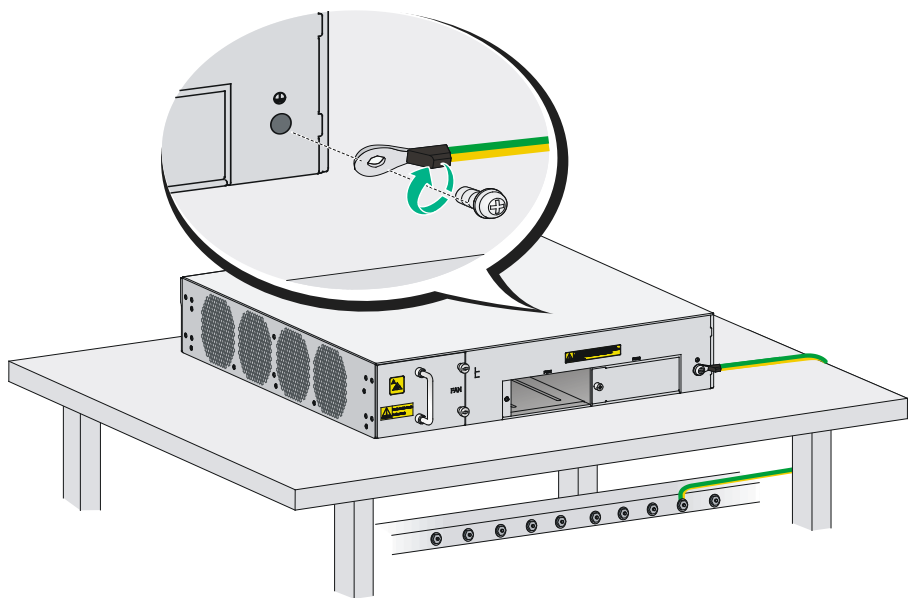
图2-8 通过接地排接地.
