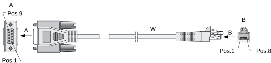
图C-1 配置口电缆示意图
