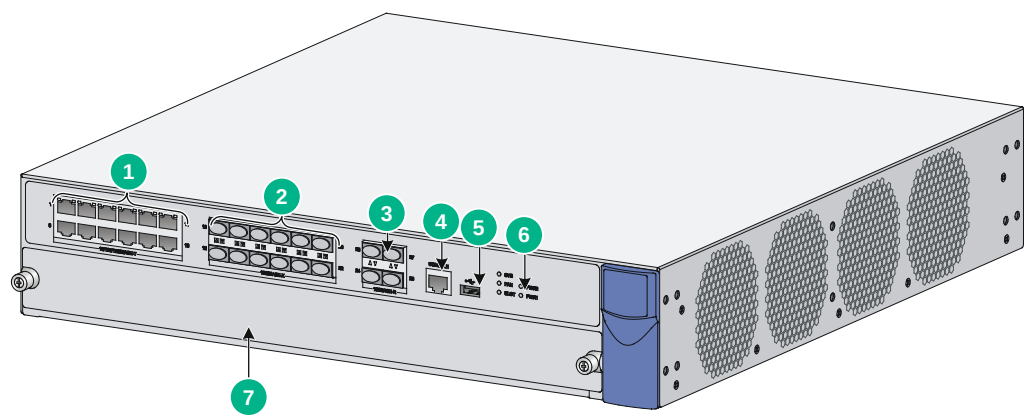
图A-1 设备前视图
