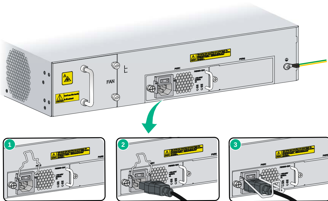
图2-15 连接交流电源线
