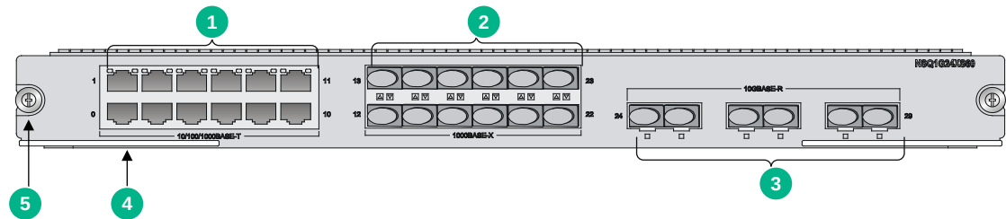
图A-3 NSQ1G24XS60 接口模块正视图
