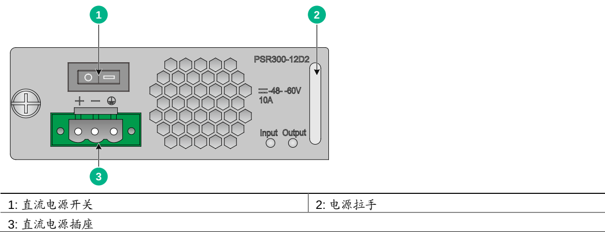
图A-5 直流电源模块外观
