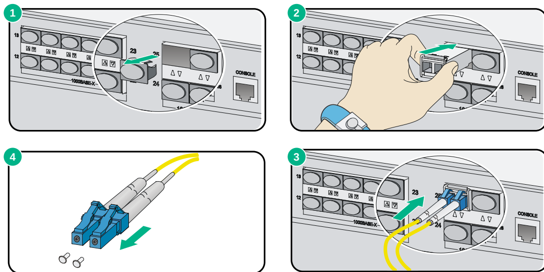
图2-14 连接光纤
