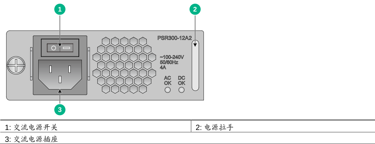
图A-4 交流电源模块外观
