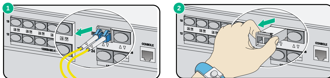
图4-4 拆卸光接口模块示意图
