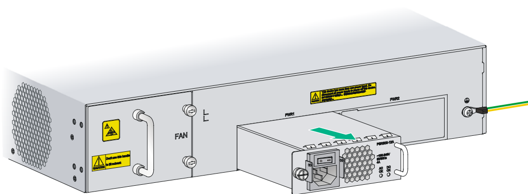
图4-1 拆卸电源模块
