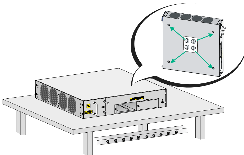
图2-2 工作台安装方式
