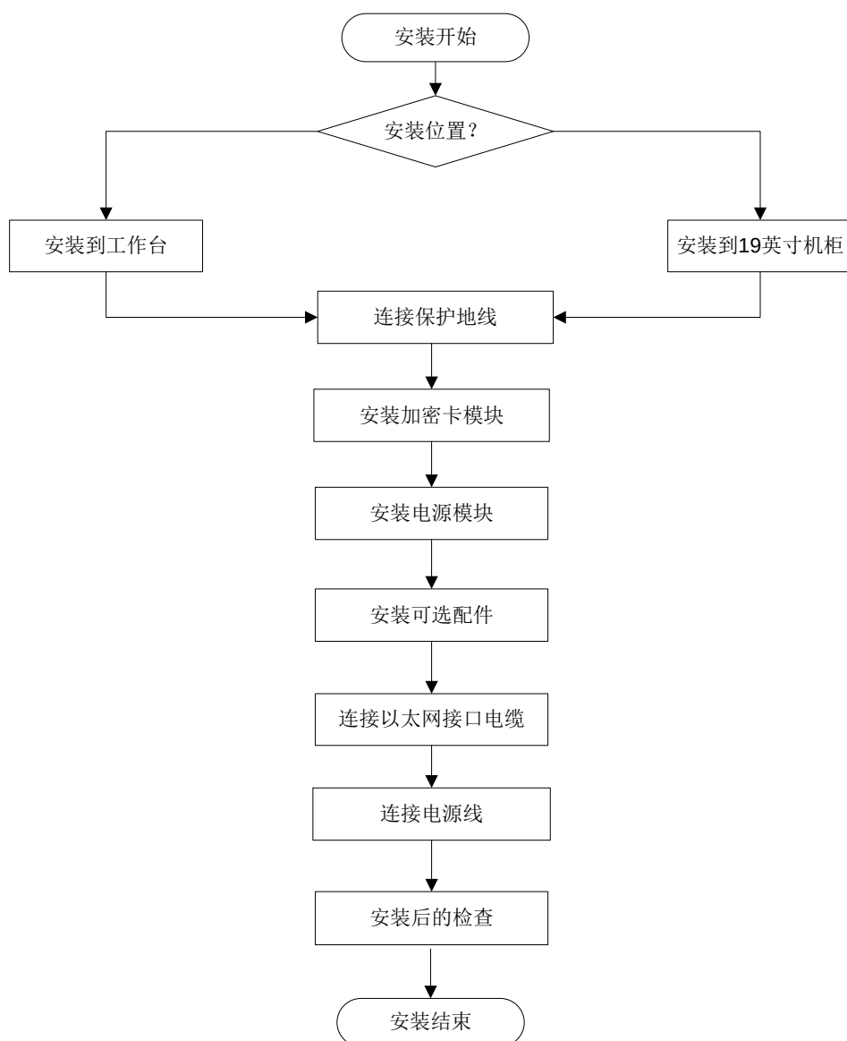
图2-1 设备安装流程示意图
