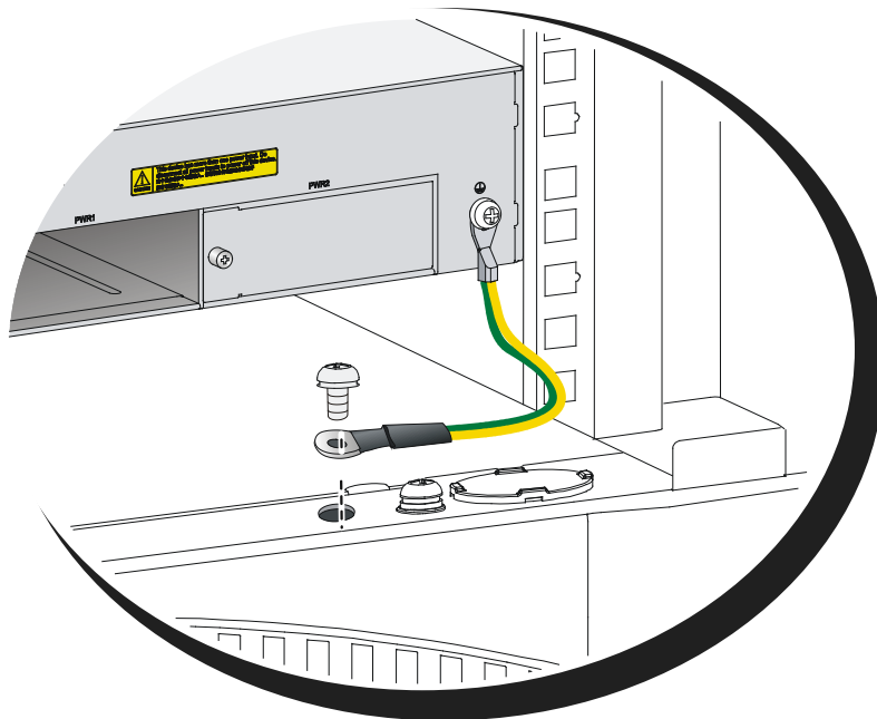
图2-7 连接到机柜接地
